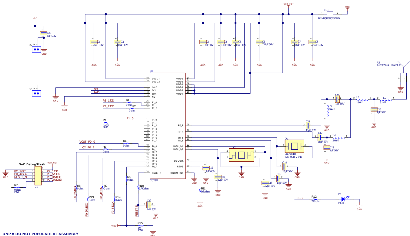
Figure 23. BLE Section
