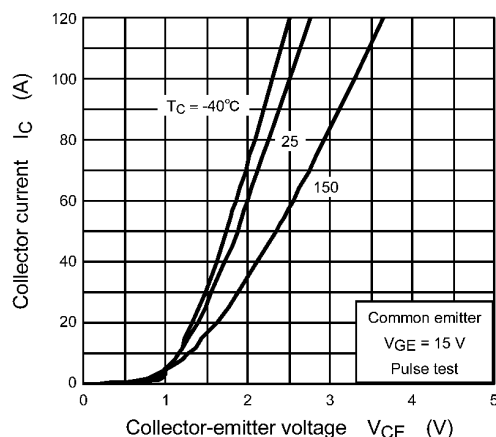
Fig. 8.4 I_C - V_{CE}
