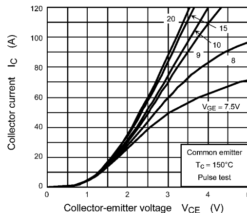
Fig. 8.3 I_C - V_{CE}
