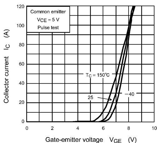
Fig. 8.6 I_C - V_{GE}
