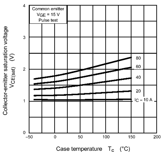
Fig. 8.5 V_{CE(sat)} - T_C
