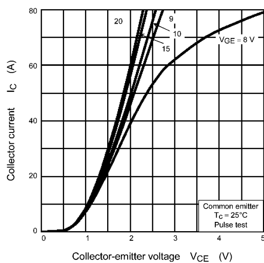
Fig. 8.2 I_C - V_{CE}
