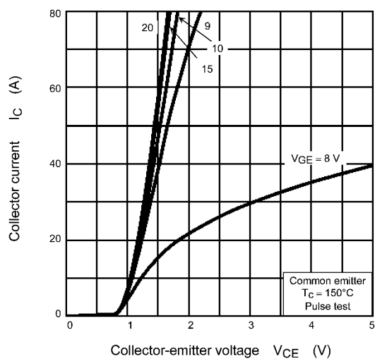
Fig. 8.3 I_C - V_{CE}
