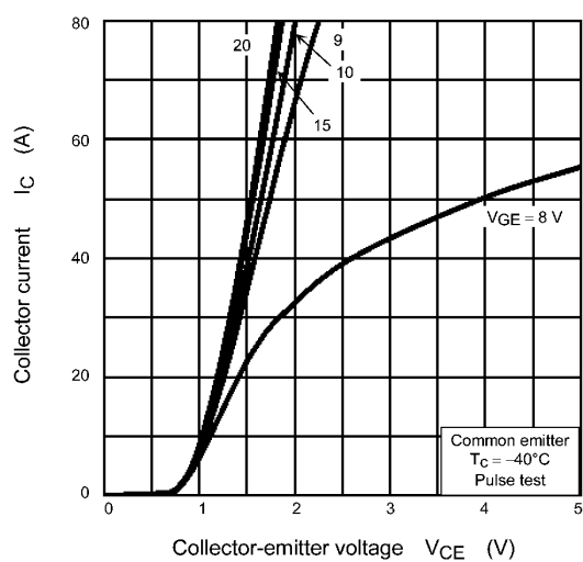
Fig. 8.1 I_C - V_{CE}
