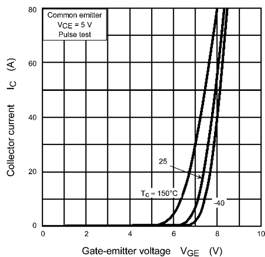
Fig. 8.4 I_C - V_{GE}
