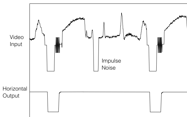
Fig. 16 Horizontal Output
