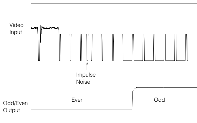
Fig. 15 Odd/Even Output
