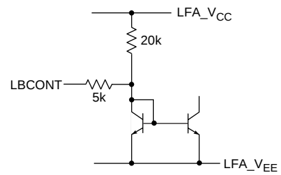
Fig. 12 LBCONT Circuit
