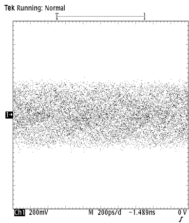
Fig. 13 Input 100m (Belden 1694A)
