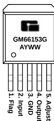
TO-263-5
