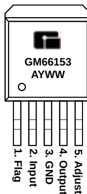
TO-263-5
