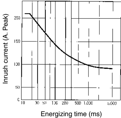
G3NE-220T(L)-(-2)(US)
