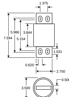
Fig. 2: 900-1000 Amp Range
