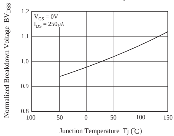
Fig3. BV_{DSS} - T_j
