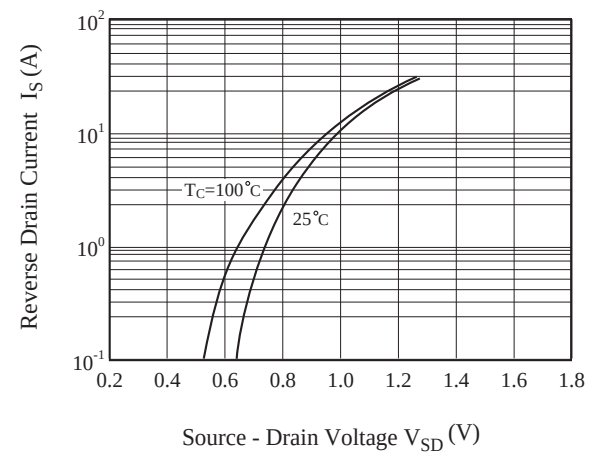
Fig5. I_S - V_{SD}
