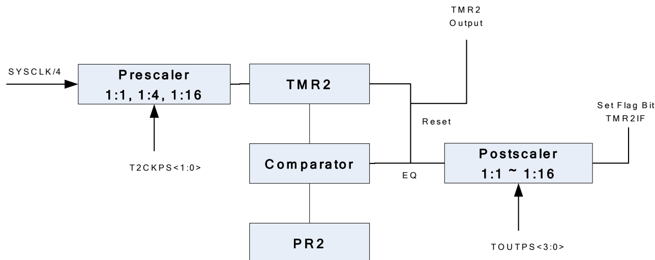
图 9.1 定时器 2 框图
