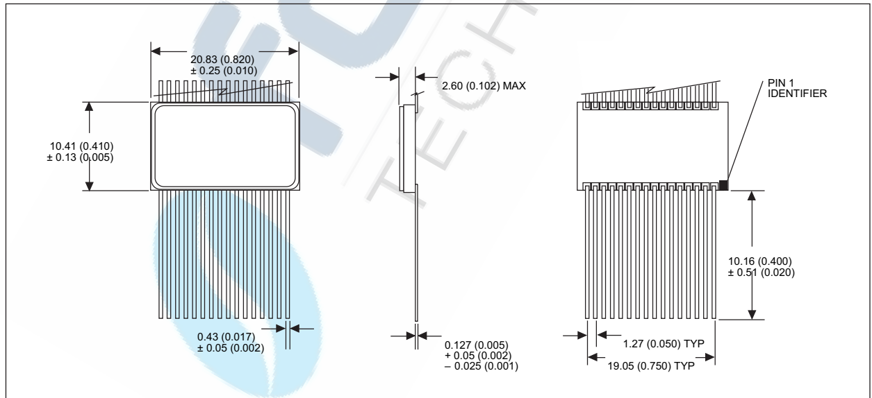
32 Pin FP
