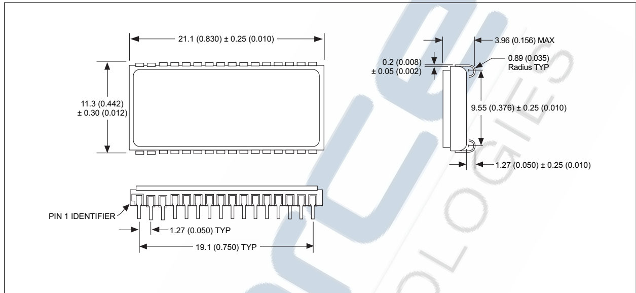
32 pin CSOJ
