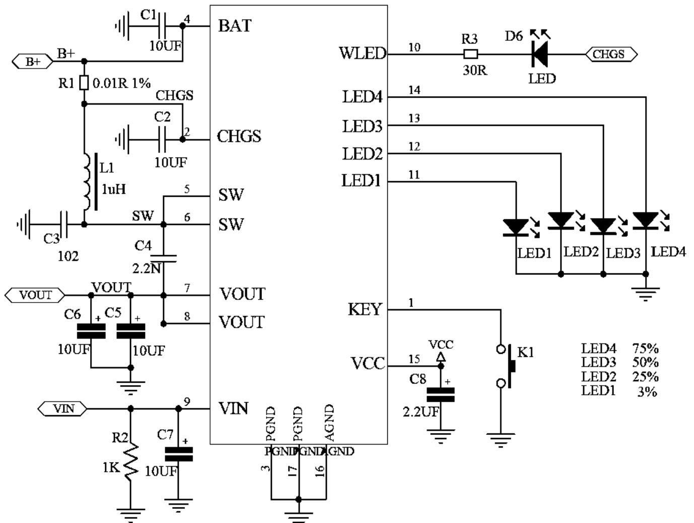
典型应用电路图
