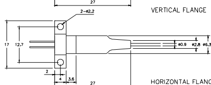
HORIZONTAL FLANGE
