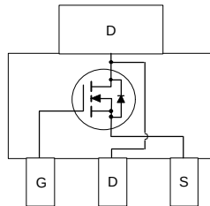
SOT-223* (J23Z)
