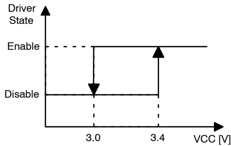
Figure 27. UVLO
