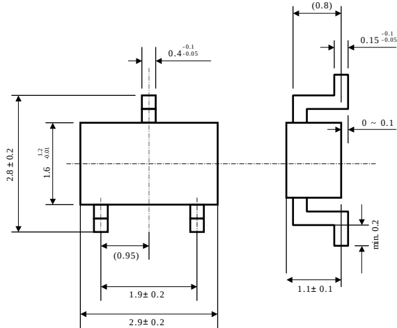
SOT-23-3:
