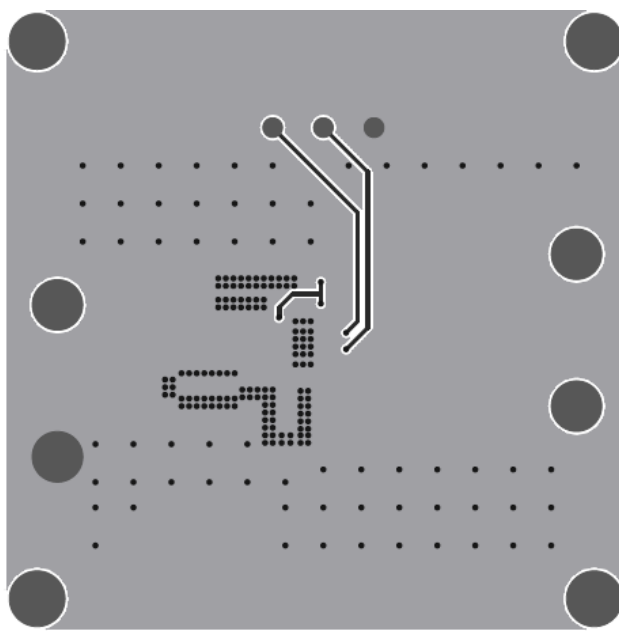
Figure 2—Bottom Layer
