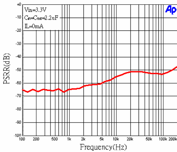
PSRR
