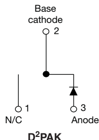
VS-ETU1506S-M3
