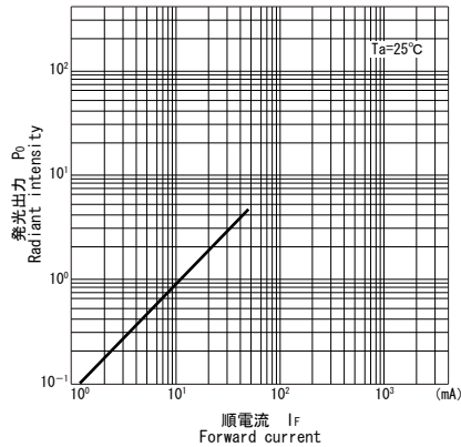
■発光出力／順電流特性 P_O/I_F
