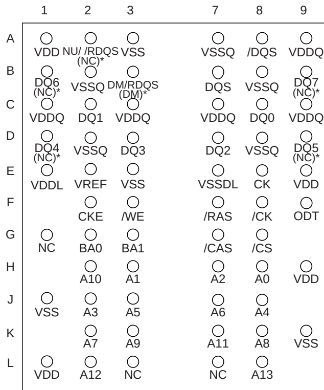
60-ball FBGA (μBGA)
