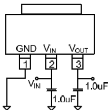
SOT89
