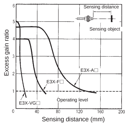
E32-D12F
