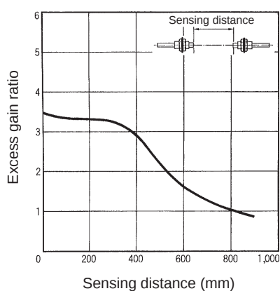
E32-T11L + E39-F1
