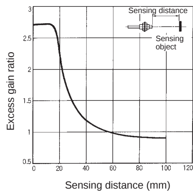
E32-D21L
