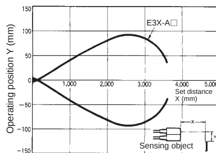
E32-R16
