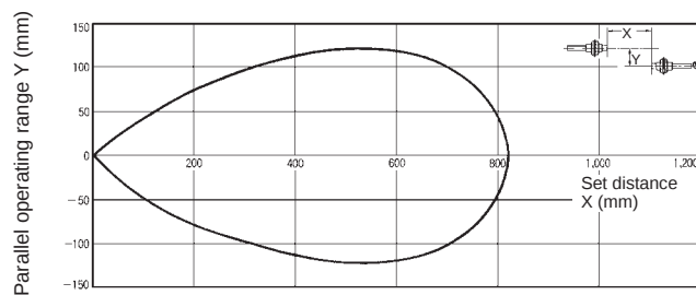
E32-T11L + E39-F2
