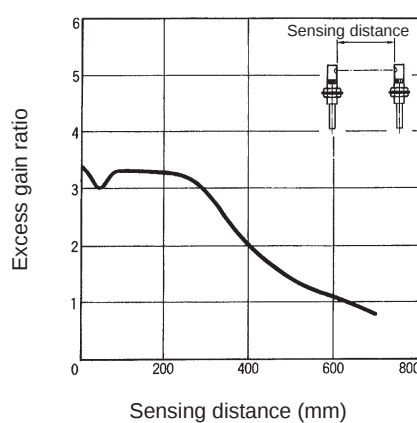
E32-T11L + E39-F2
