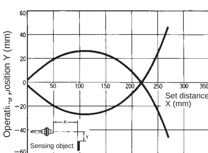
E32-D33
