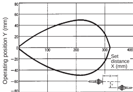
E32-T21
