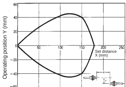
E32-T14
