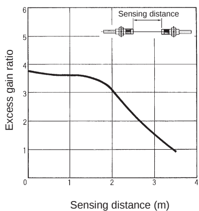
E32-T11L + E39-F1
