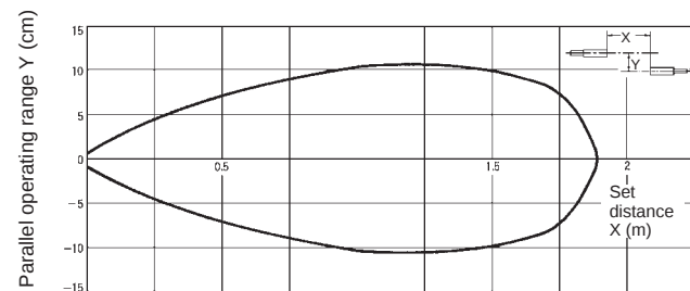
E32-T12F
