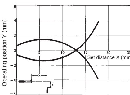
E32-T84S
