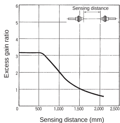
E32-T11L + E39-F3
