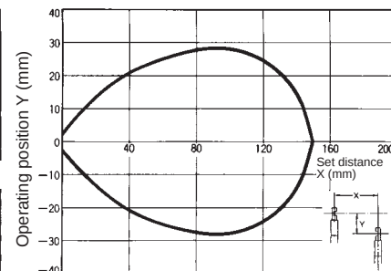
E32-T12F
