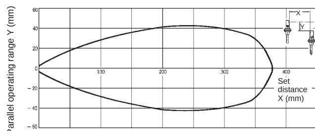
E32-T14L
