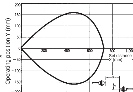
E32-T24
