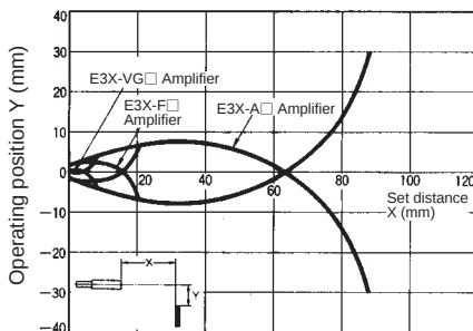
E32-D32L
