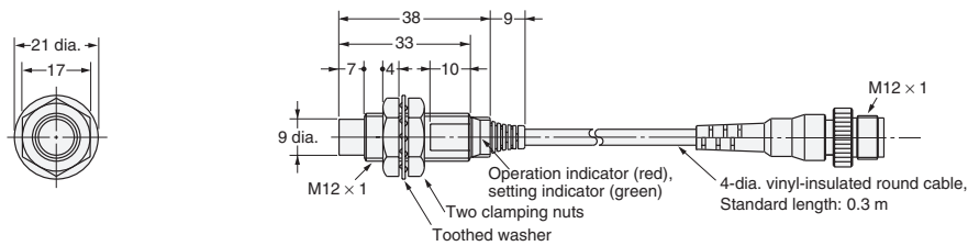
Fig. 32: E2E-X7D1-M1GJ E2E-X7D1-M1J-T
