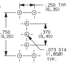
E101MD1_BE SPDT
