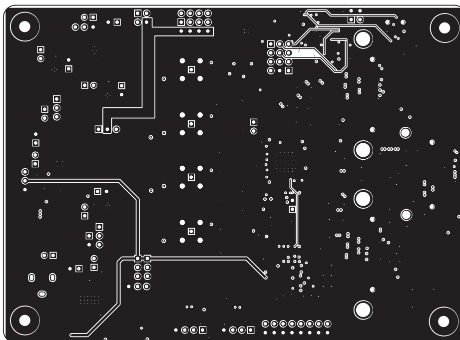
Figure 3-4. Layer 2
