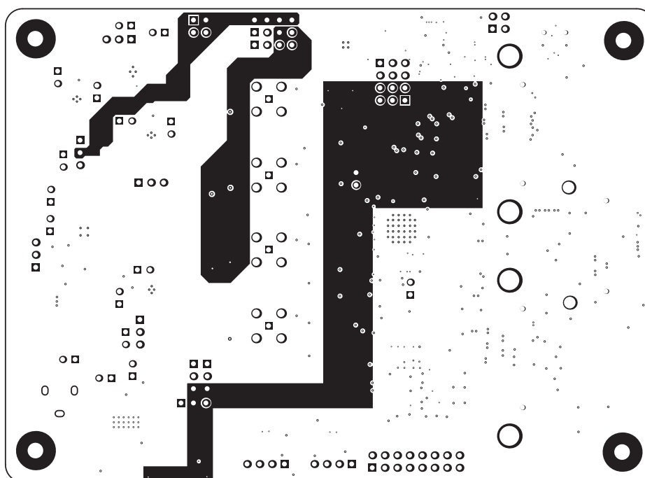
Figure 3-6. Layer 4
