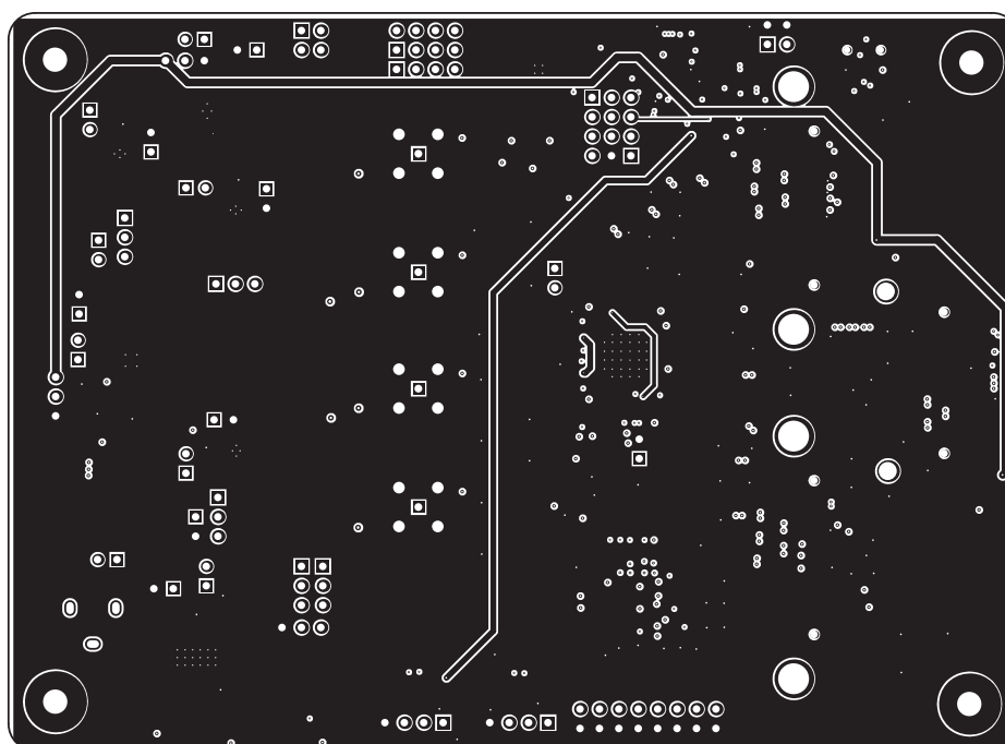
Figure 3-7. Layer 5
