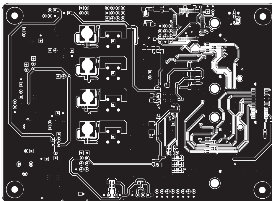
Figure 3-8. Bottom Layer 6
