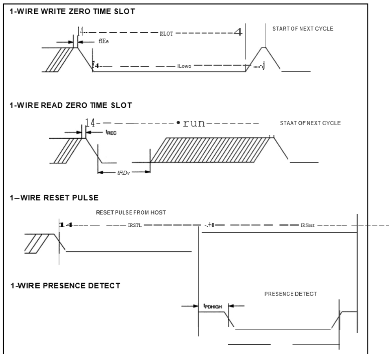
图 18. 时序
