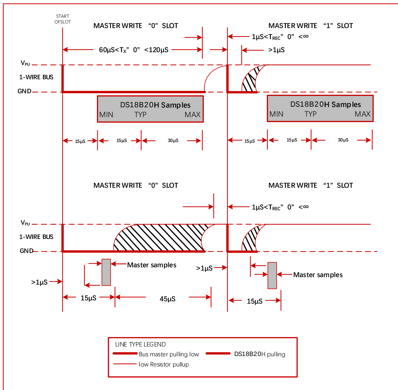
图 14. 读/写时序图
