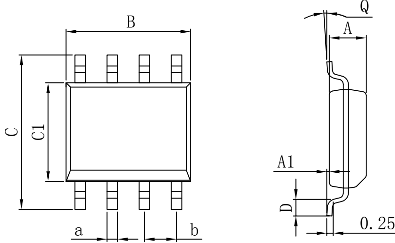
SOP8
