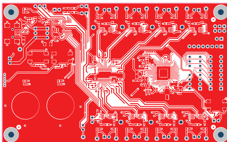
Figure 16. Top Layer
