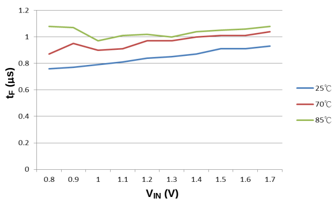
t_F vs. V_{IN} ( V_{BIAS}=3.2V )
