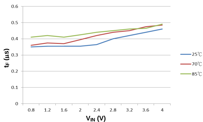
t_F vs. V_{IN} ( V_{BIAS}=5.5V )
