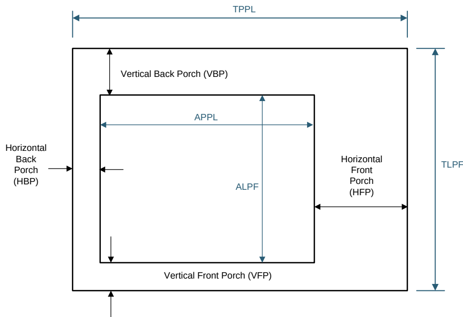
Figure 18. Timing Parameter Diagram
