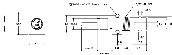
ST Receptacle
