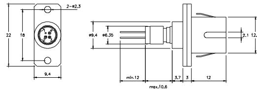
SC Receptacle
