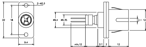
SC Receptacle
