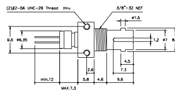
ST Receptacle
