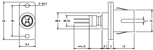
SC Receptacle
