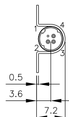
Horizontal Flange
