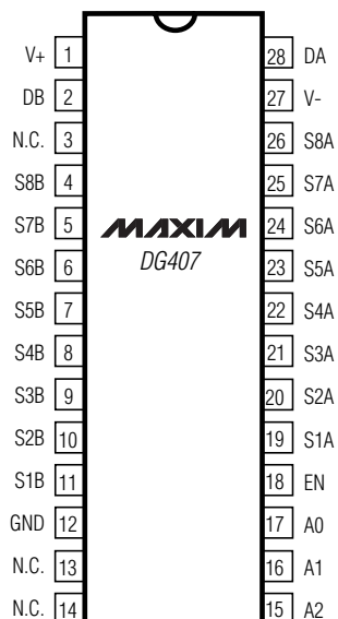
DIP/SO
