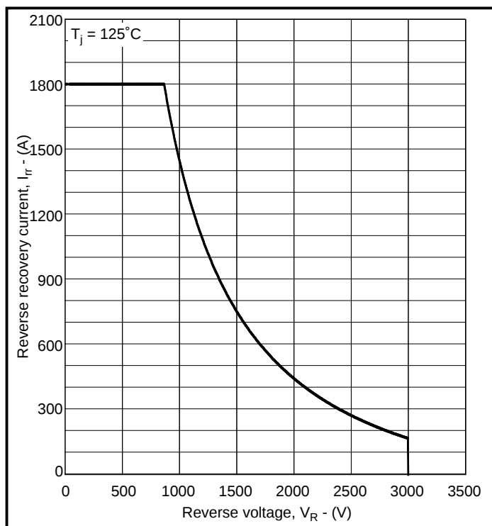
Fig. 7 RBSOA
