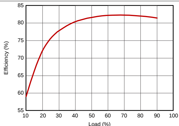
DCV010505D
