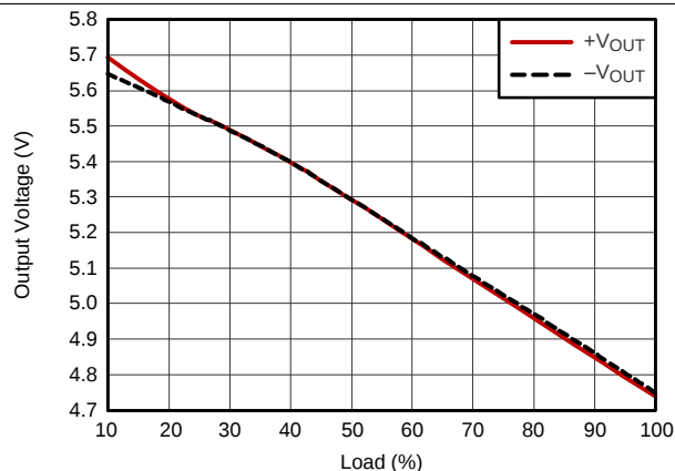
DCV010505D
