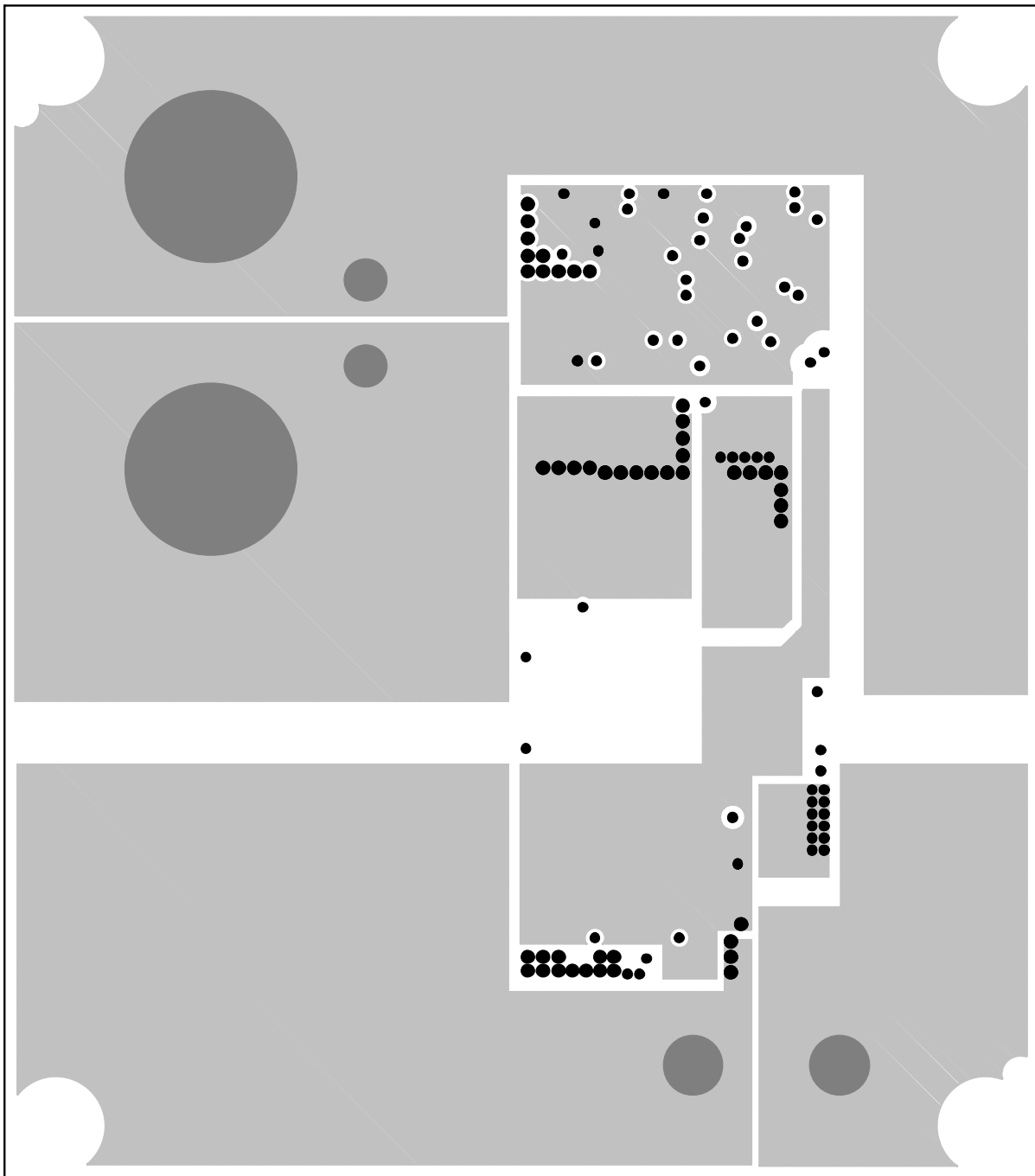
Figure 19. Layer 5
