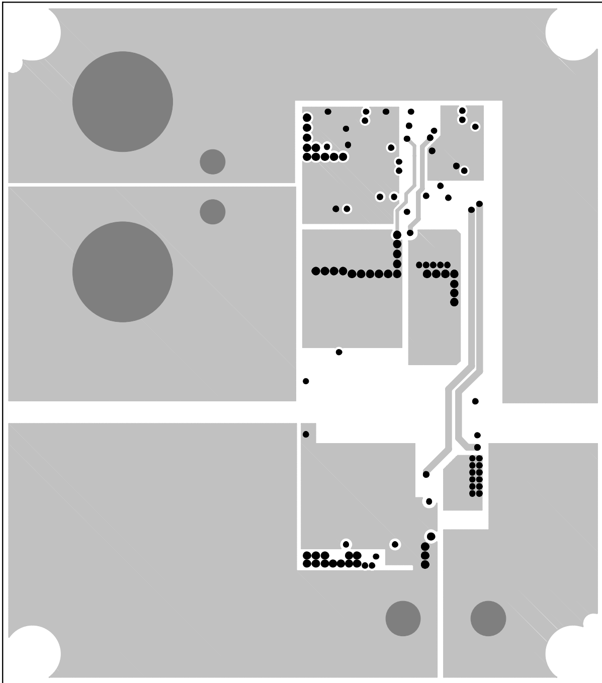
Figure 18. Layer 4
