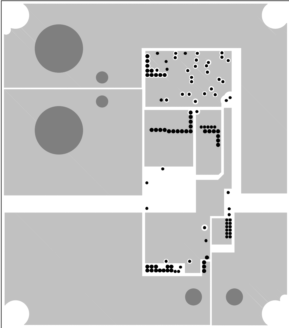
Figure 19. Layer 5
