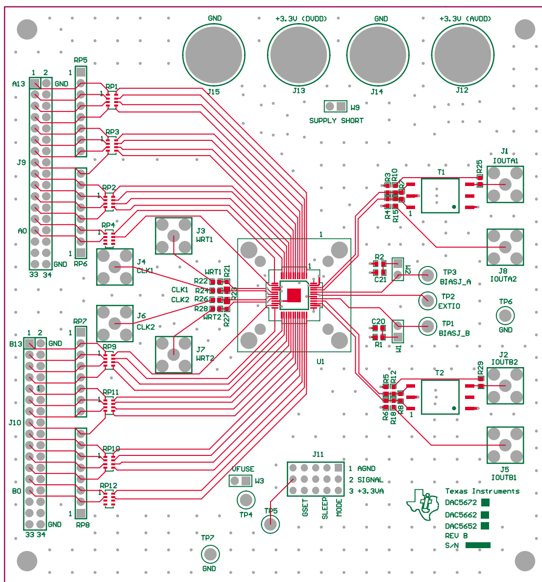
Figure 27. Top Layer 1
