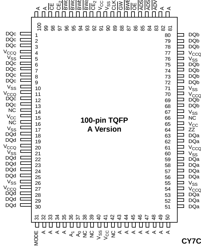
CY7C1361A 256K x 36 100-pin TQFP
