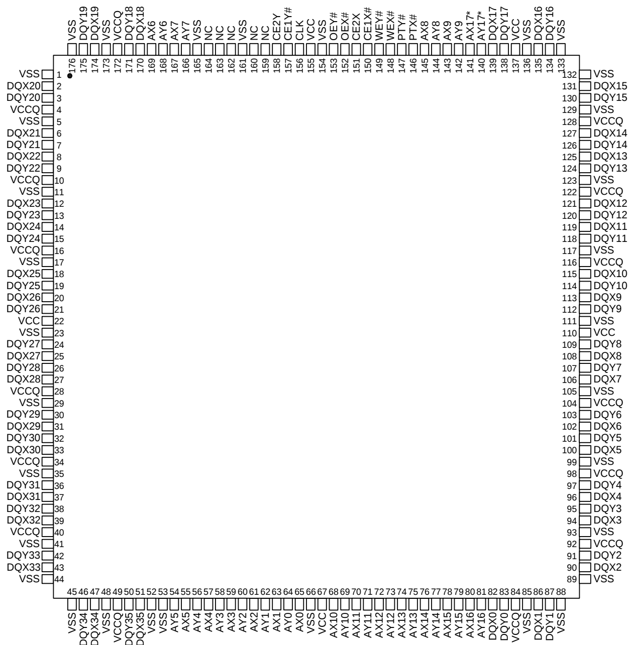
176-pin TQFP
