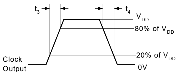
Figure 4. ER = (0.6 \times V_{DD})/t_3 , EF = (0.6 \times V_{DD})/t_4
