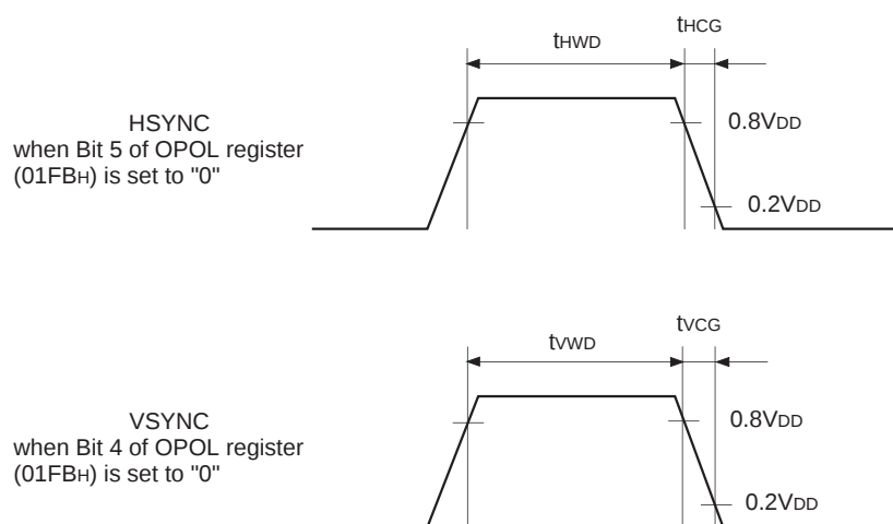
Fig. 11. OSC timing
