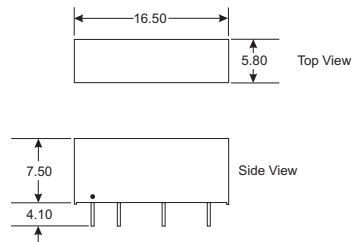
CTDD1605SF-SU1K-1 Package
