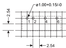
CTDD1605SF-SU1K-1 Footprint
