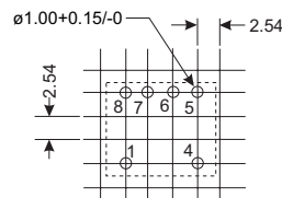
CTDD1210DF-TU1K-1 Footprint
