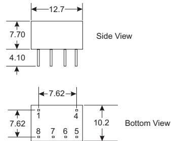
CTDD1210DF-TU1K-1 Package
