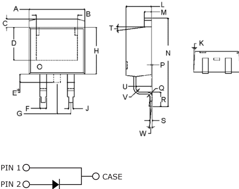
Package TO-263-2
